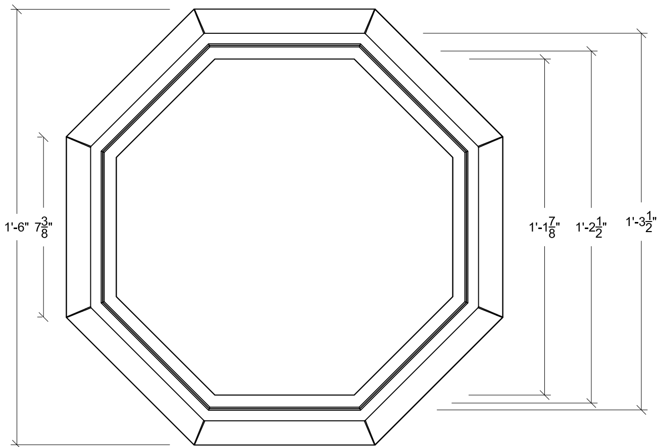
Plan view SCALE: 3"=1'-0"
